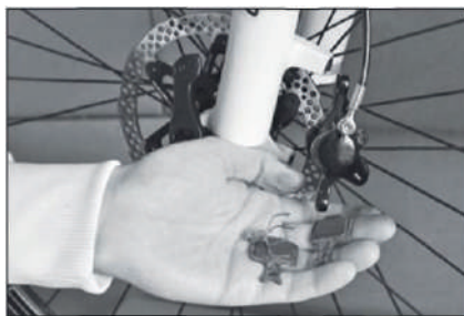
Wymienić zużyte klocki hamulcowe
