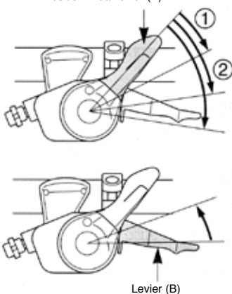
Levier (B)
