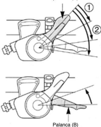
fig. 19 Posición inicial palanca (A)
